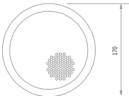
Frontansicht
