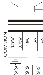
Leistungsanschlussbelegung
